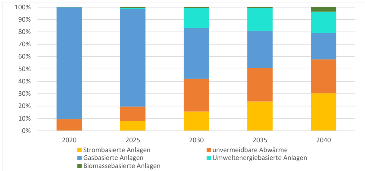
Abbildung 44: Geplante Transformation der Thüringer Fernwärmeversorgung bis 2040 gemäß den Anteilen an der Wärmemenge (n=31) 221
