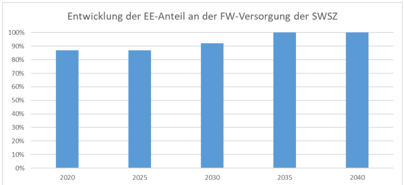
Abbildung 32 Entwicklung der EE-Anteile an der FW-Versorgung der Stadtwerke Suhl/Zella-Mehlis GmbH für das Gesamtnetz
