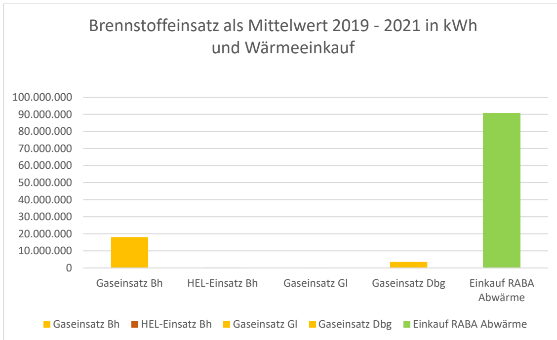
Abbildung 28 Brennstoffeinsatz und Wärmeeinkauf
