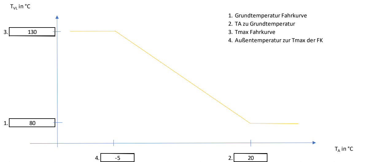
Abbildung 27 Prinzipielles Beispiel einer Temperaturfahrkurve
